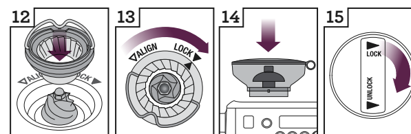
Pousser la meule supérieure en place Verrouiller la meule supérieure Insérer la trémie Verrouiller la trémie
