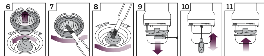
Retirer la meule supérieure Nettoyer la meule supérieure avec la brosse Nettoyer la meule inférieure avec la brosse Retirer l'hélice de tassage avec l'aimant Nettoyer la sortie de mouture avec la brosse Replacer l'hélice de tassage avec l'aimant
